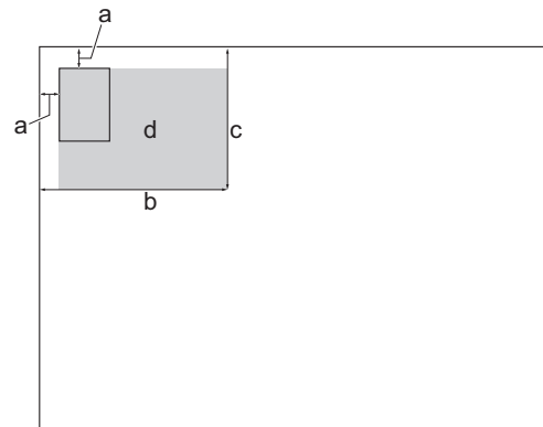
2 in 1 -henkilökorttitoiminto (vaaka)
